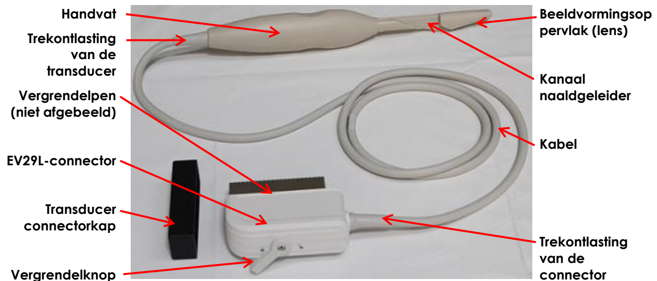
Afbeelding 1: ExactVu EV29L-transducer
