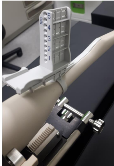
Afbeelding 21: EV29L met ingestoken EV29L steriele transperineale naaldgeleider (zonder huls afgebeeld)
